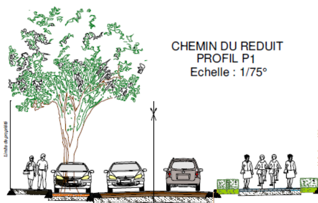
Coupe de la rue du Réduit : requalification de la voirie, aménagement paysager, création d'une voie verte séparée par un terre-plein latéral. © Bordeaux Métropole
